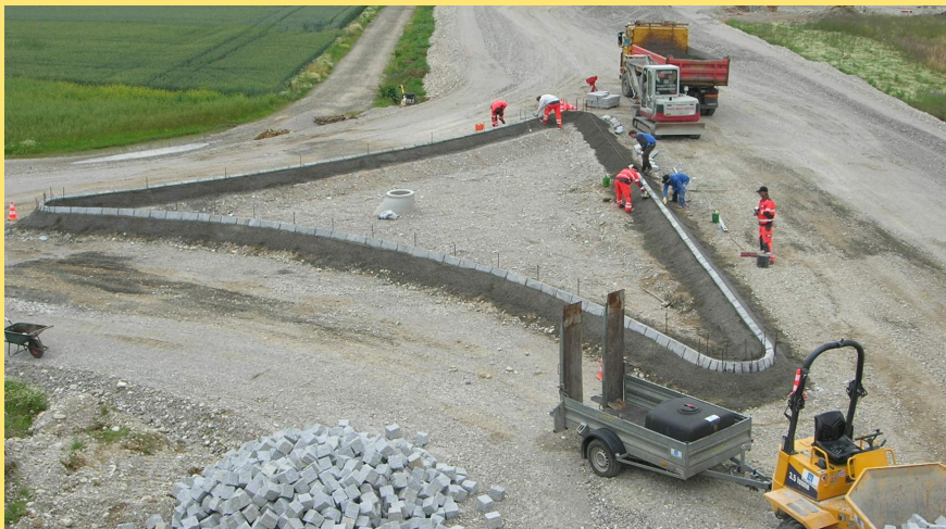
(Abb.: Versetzen von Leistensteinen im Bereich des Anschlusses Hargelsberg Nord)
