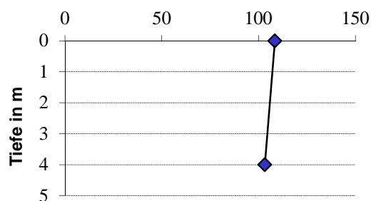
Almsee O 2 -Sättigung % Mittelwerte 2007 - 2012
