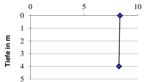
Almsee pH-Wert Mittelwerte 2007 - 2012
