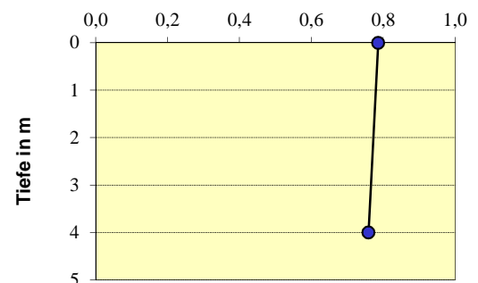
Almsee DOC mg/l Mittelwerte 2007 - 2012
