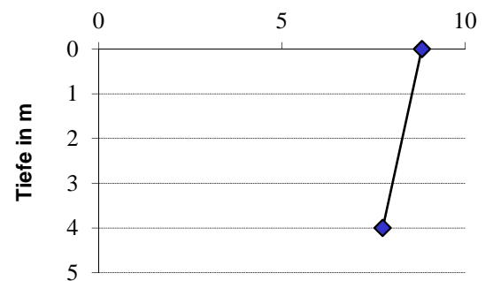
Almsee Temperatur °C Mittelwerte 2007 - 2012
