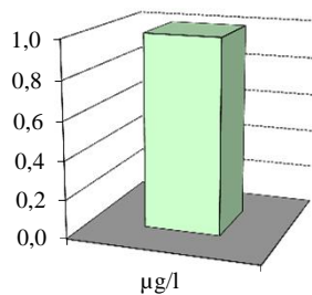
Almsee Chlorophyll-a Mittelwert 11/2007-2012
