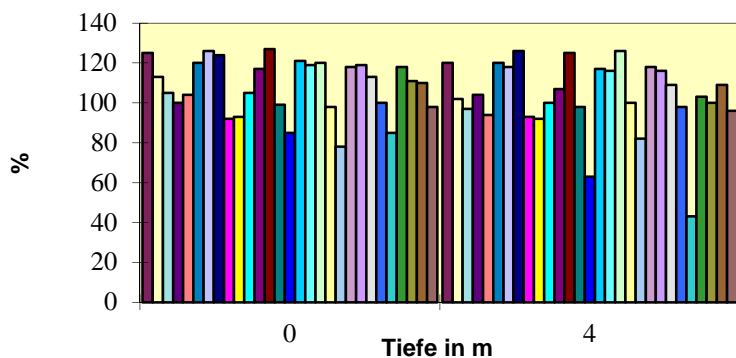
Almsee O 2 -Sättigung (2007-2012)
