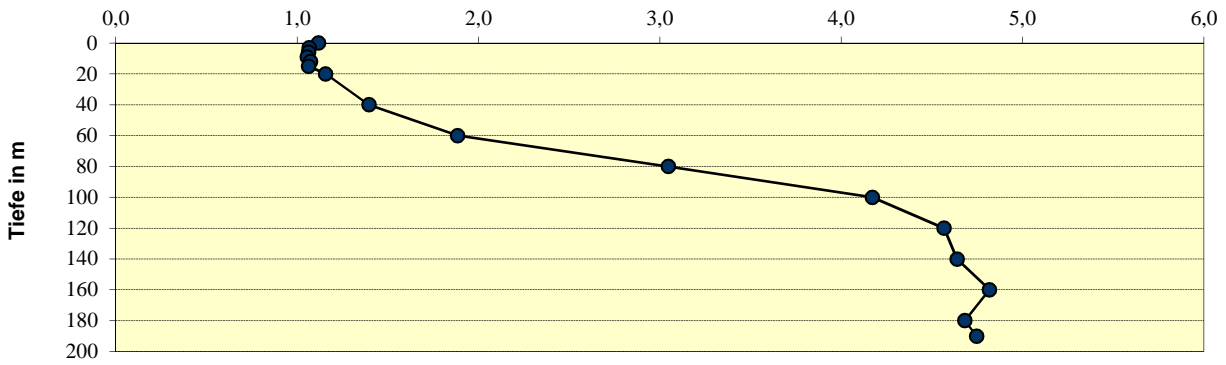
Traunsee-Mitte Kalium Mittelwerte mg/l
