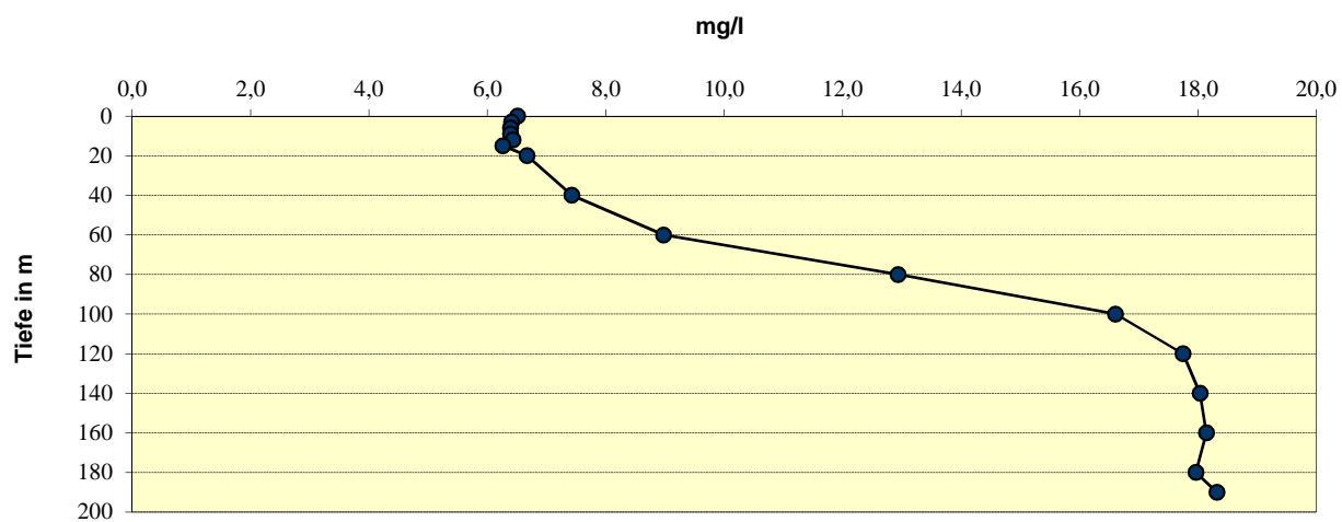
Traunsee-Mitte SO 4 Mittelwerte
