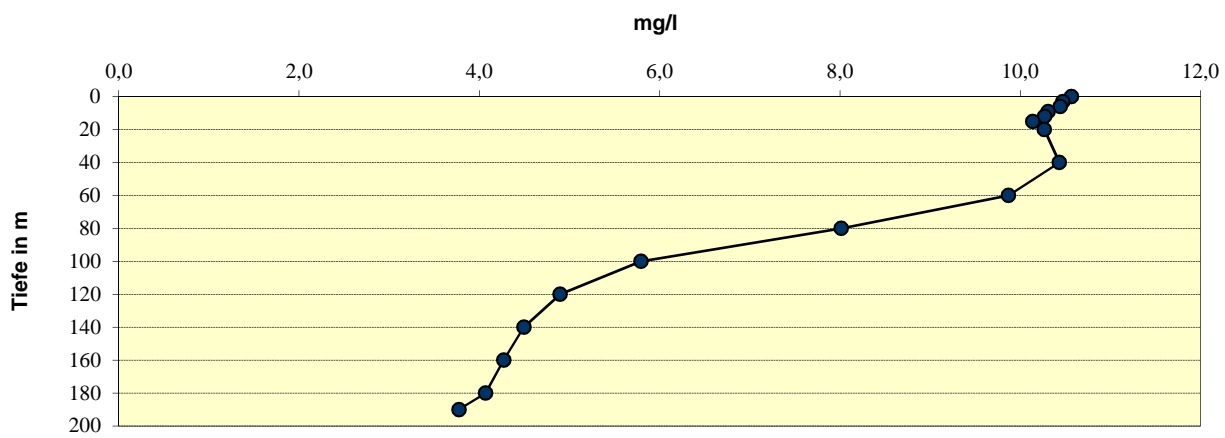
Traunsee-Mitte O 2 -sofort Mittelwerte
