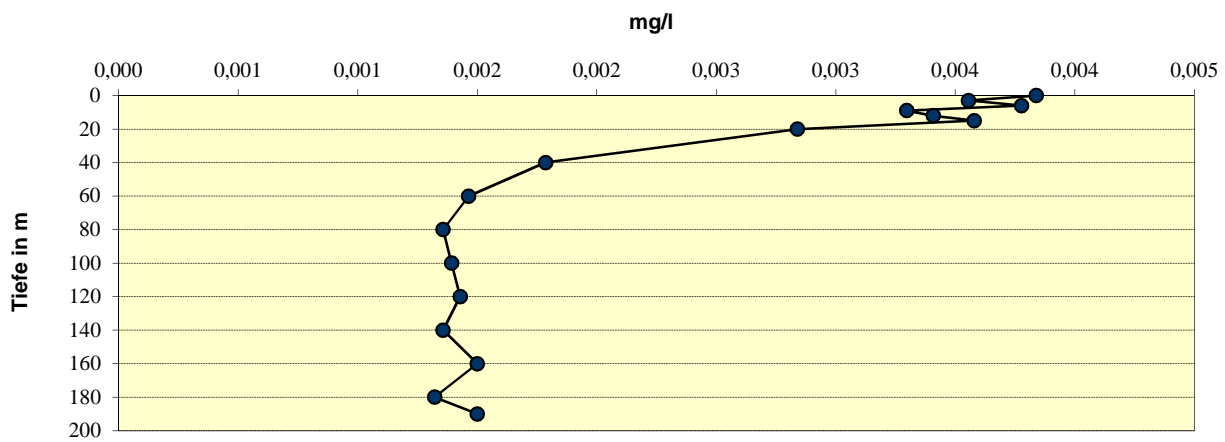
Traunsee-Mitte NO2-N Mittelwerte
