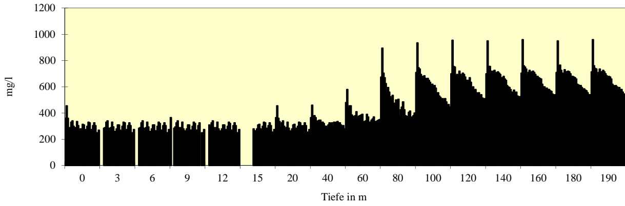
Traunsee-Mitte Leitfähigkeit
