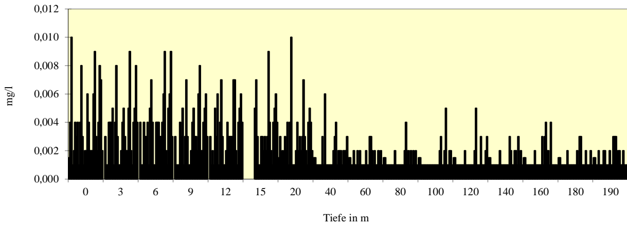
Traunsee-Mitte NO2-N
