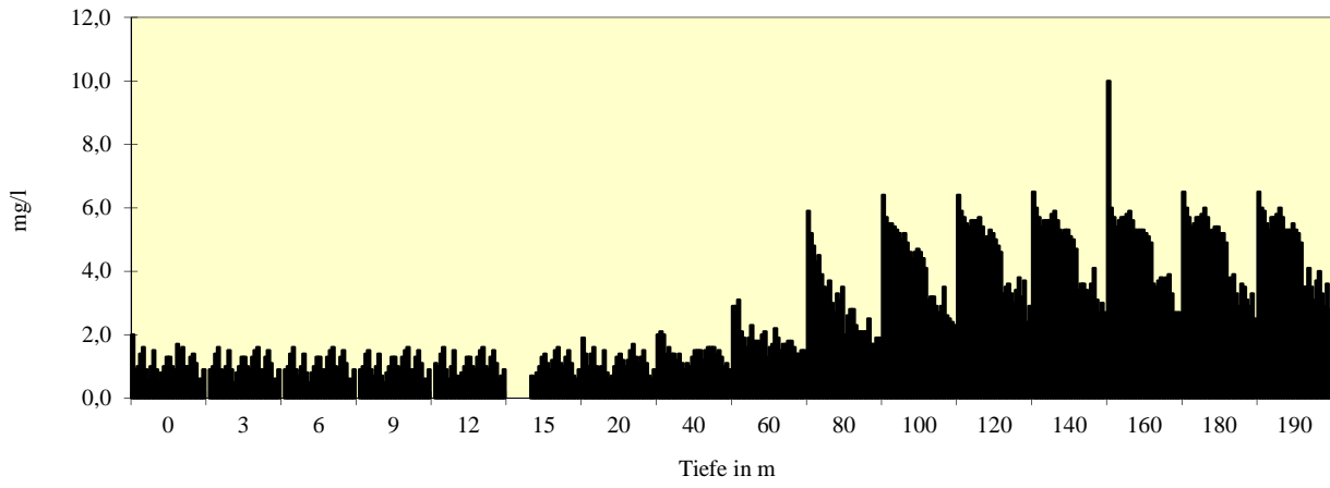
Traunsee-Mitte Kalium
