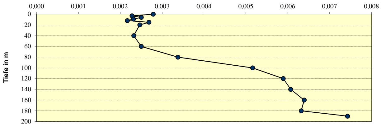
Traunsee-Mitte Ges. P-filtriert Mittelwerte mg/l
