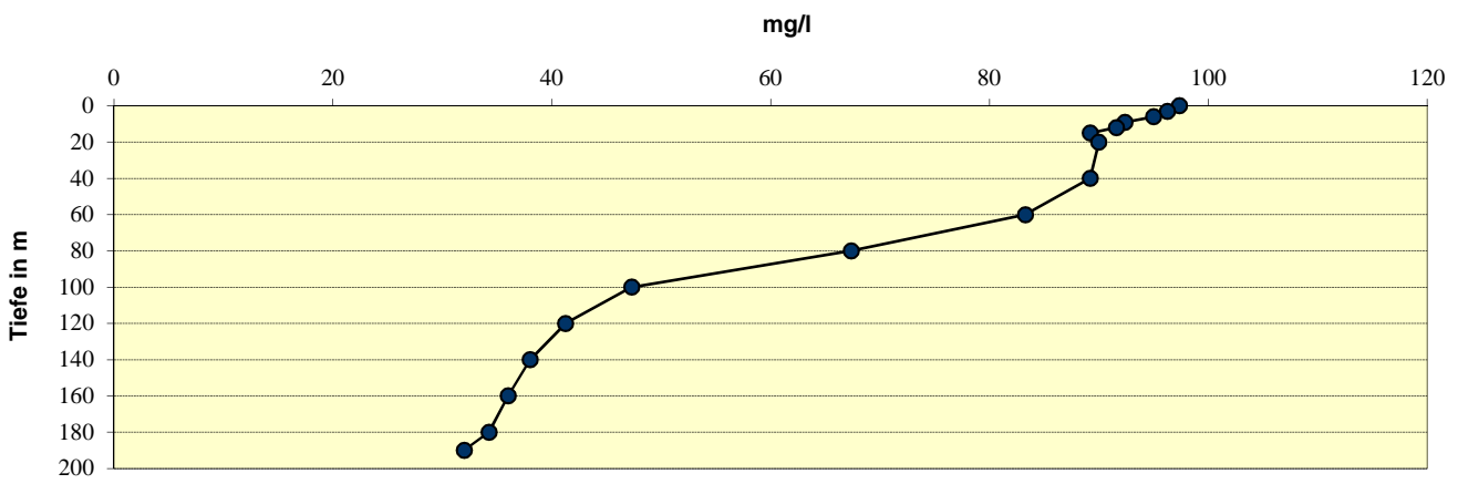
Traunsee-Mitte O 2 -Sättigung Mittelwerte
