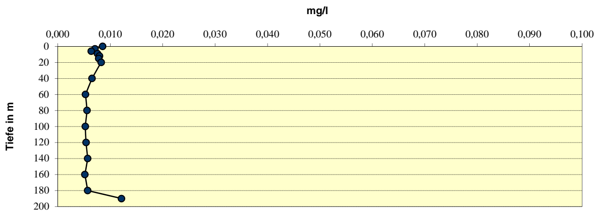
Traunsee-Mitte NH4-N Mittelwerte
