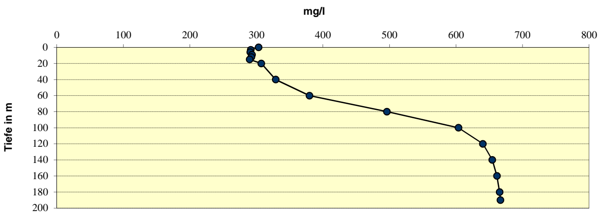
Traunsee-Mitte Leitfähigkeit Mittelwerte
