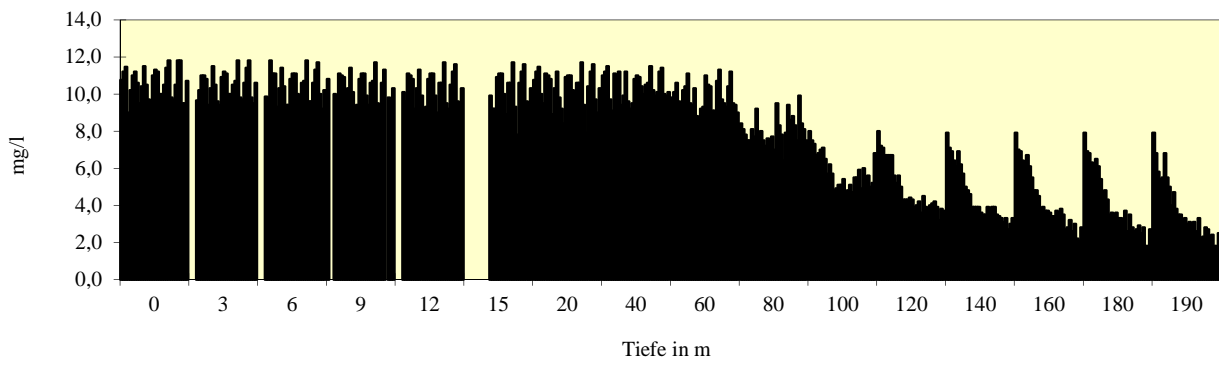
Traunsee-Mitte O 2 -sofort Mittelwerte
