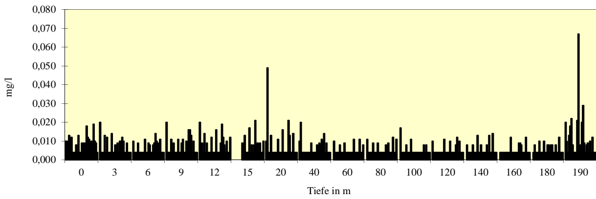
Traunsee-Mitte NH4-N
