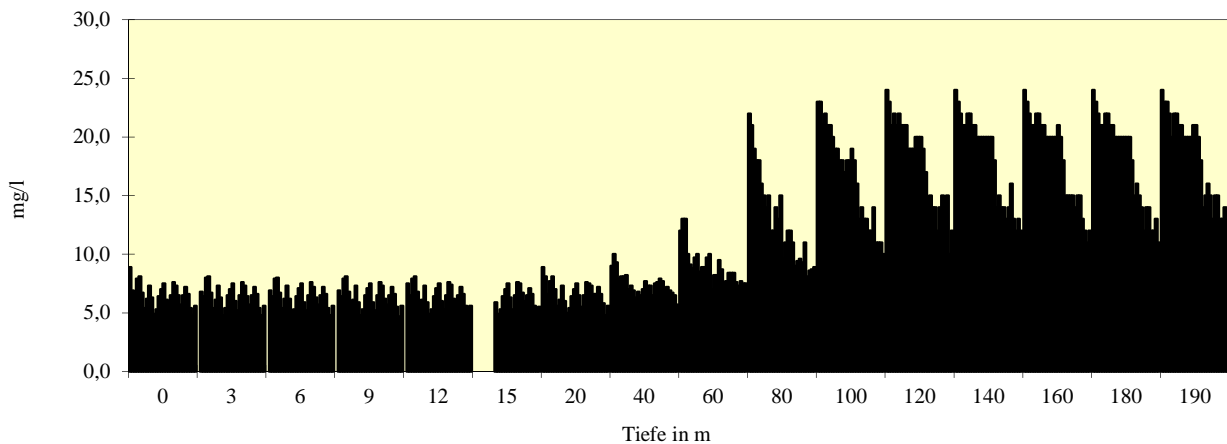
Traunsee-Mitte SO 4
