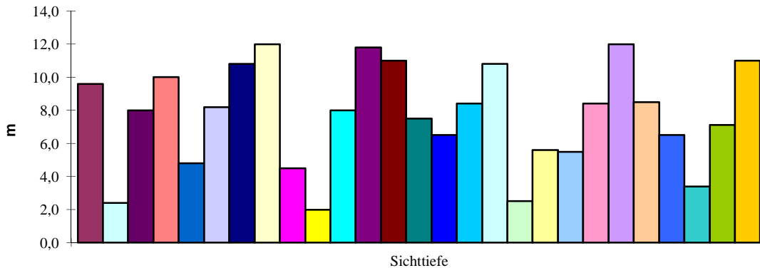
Traunsee-Mitte Sichttiefe
